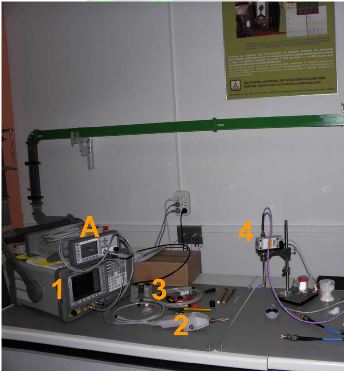
Figura 3. Unitatea de baza a analizorului de spectru (1) sonda pentru masurarea de prezie a puterii de intrare (2) conectata si la un powermetru existent (A), mixerele de inalta frecventa (3) si modulul de calibrare E-Cal (4).
